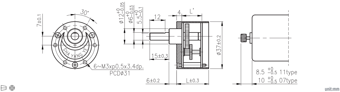
外形尺寸 & 馬達齒鉋合尺寸 / Appearance Size & Pinion Assembly Dimension
