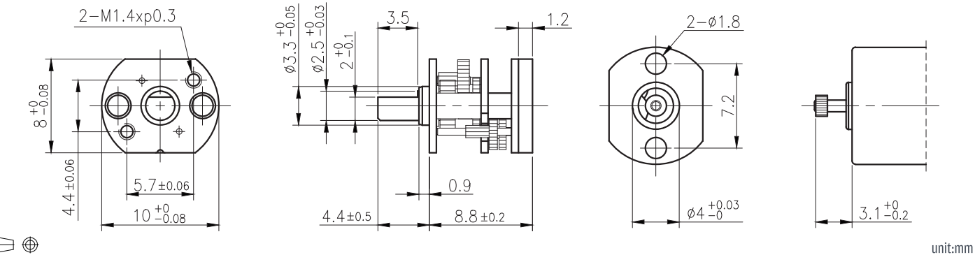
外形尺寸 & 馬達齒鉋合尺寸 / Appearance Size & Pinion Assembly Dimension
