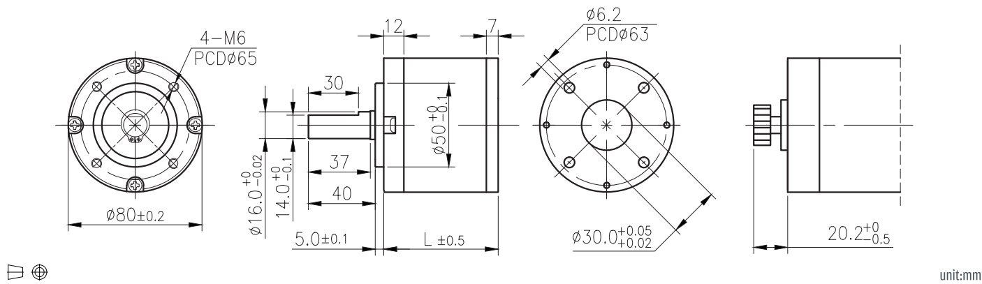
外形尺寸 & 馬達齒鉋合尺寸 / Appearance Size & Pinion Assembly Dimension
