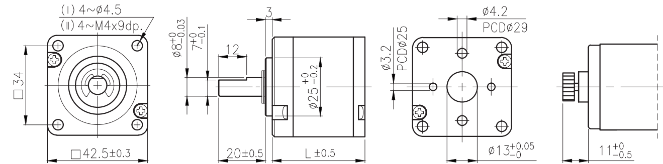
外形尺寸 & 馬達齒鉋合尺寸 / Appearance Size & Pinion Assembly Dimension
