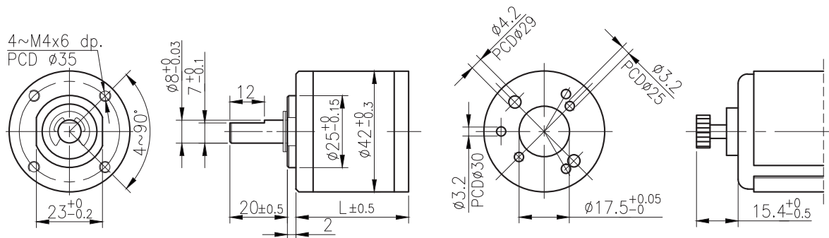
外形尺寸 &amp; 馬達齒鉚合尺寸 / Appearance Size &amp; Pinion Assembly Dimension
