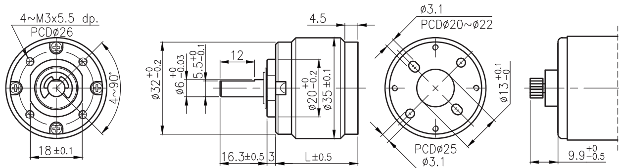
外形尺寸 &amp; 馬達齒鉋合尺寸 / Appearance Size &amp; Pinion Assembly Dimension
