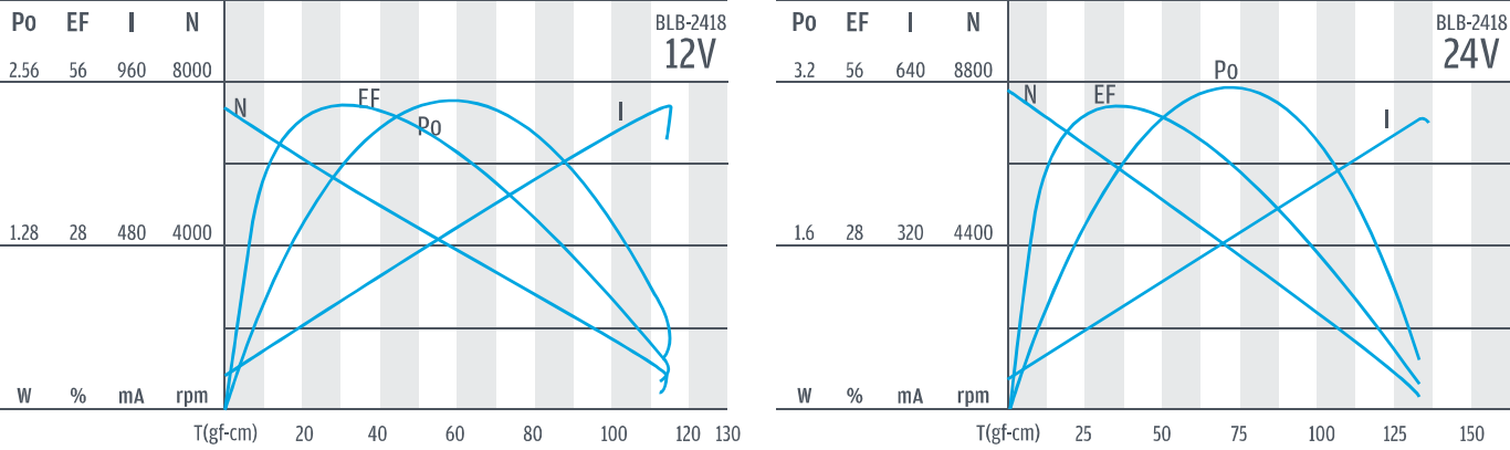
馬達單體特性/Motor Characteristics
