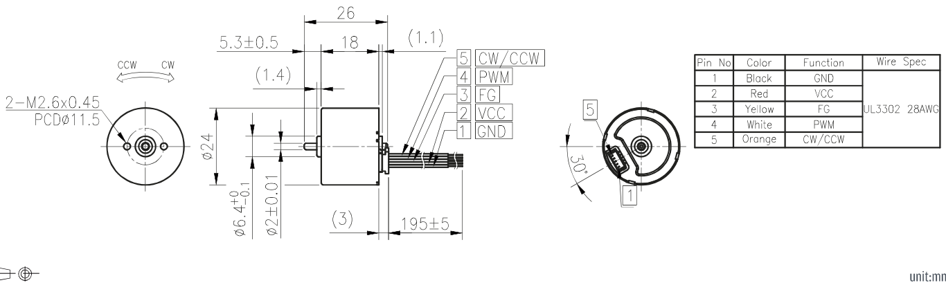
馬達單體型式/Motor Data
