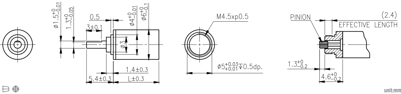
外形尺寸 & 馬達齒鉚合尺寸 / Appearance Size & Pinion Assembly Dimension
