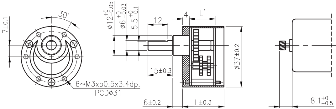
外形尺寸 & 馬達齒鉋合尺寸 / Appearance Size & Pinion Assembly Dimension
