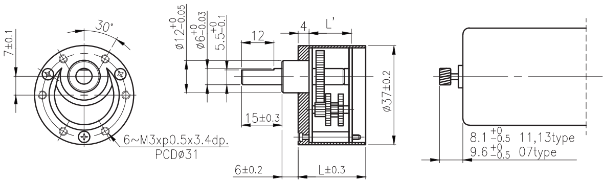
外形尺寸 & 馬達齒鉋合尺寸 / Appearance Size & Pinion Assembly Dimension
