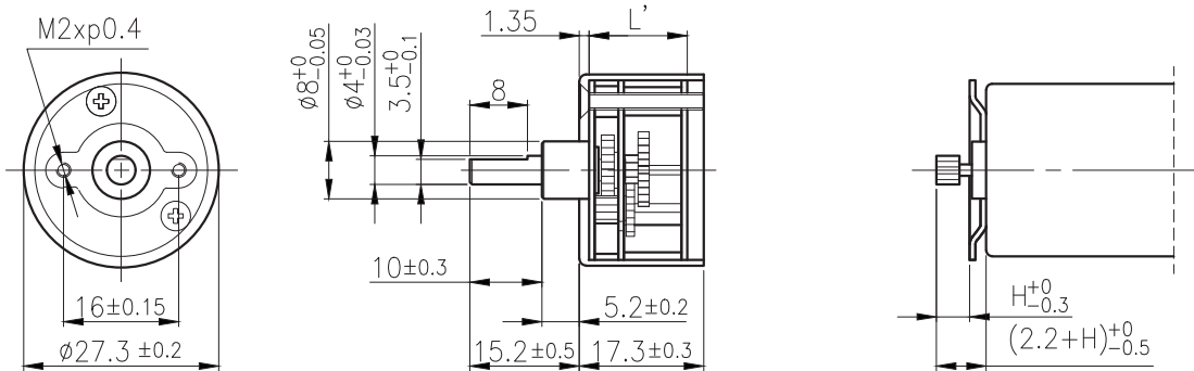
外形尺寸 & 馬達齒鉚合尺寸 / Appearance Size & Pinion Assembly Dimension
