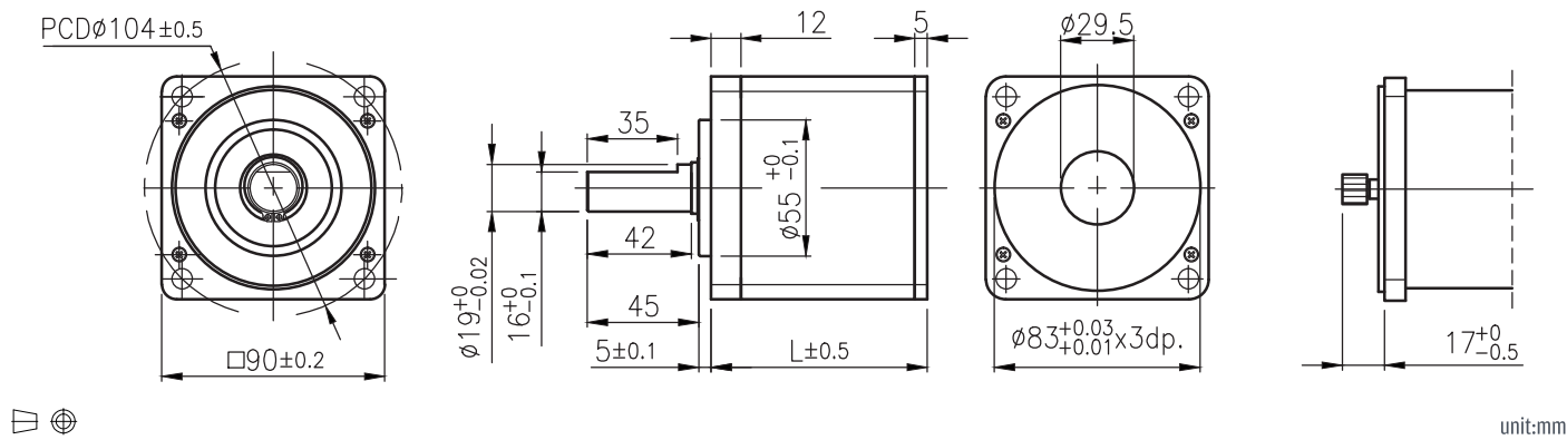
外形尺寸 & 馬達齒鉚合尺寸 / Appearance Size & Pinion Assembly Dimension
