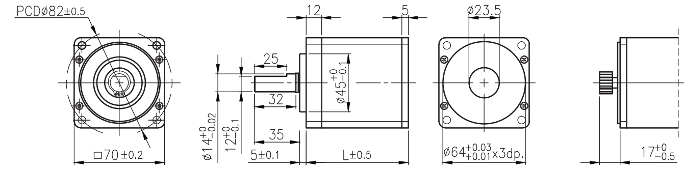
外形尺寸 & 馬達齒鉚合尺寸 / Appearance Size & Pinion Assembly Dimension
