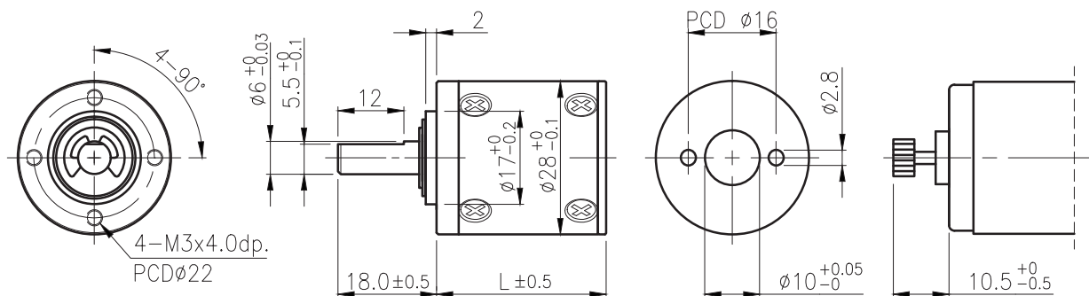
外形尺寸 &amp; 馬達齒鉚合尺寸 / Appearance Size &amp; Pinion Assembly Dimension
