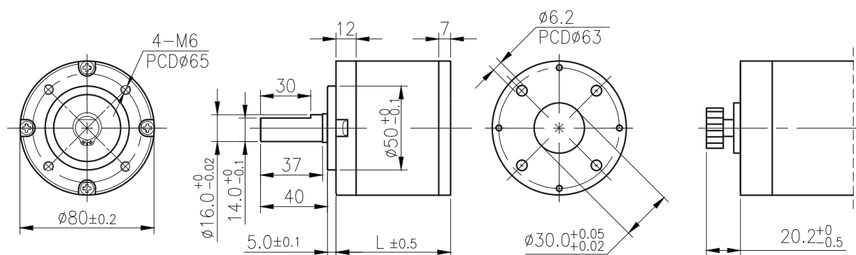
外形尺寸 & 馬達齒鉚合尺寸 / Appearance Size & Pinion Assembly Dimension
