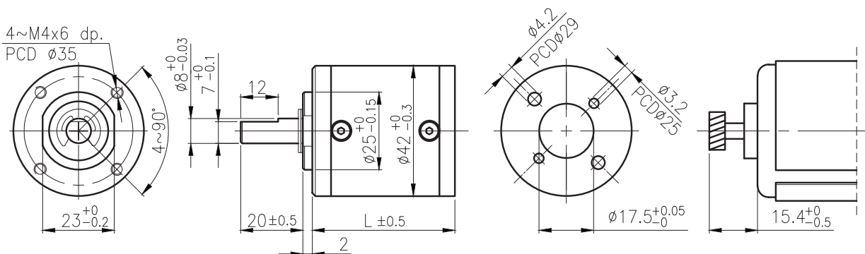
外形尺寸 & 馬達齒啮合尺寸 / Appearance Size & Pinion Assembly Dimension
