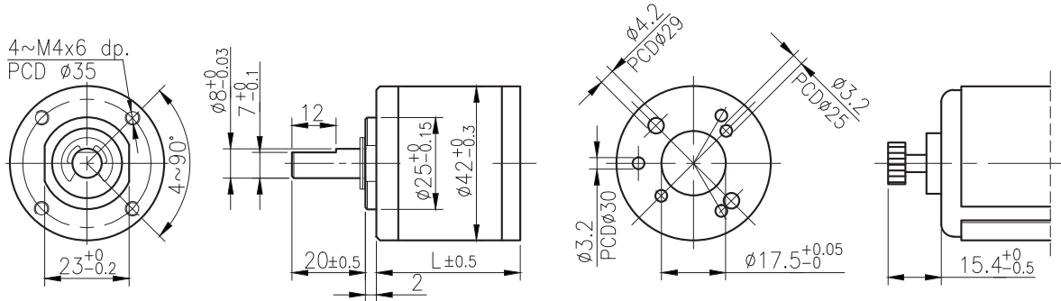
外形尺寸 & 馬達齒腳合尺寸 / Appearance Size & Pinion Assembly Dimension
